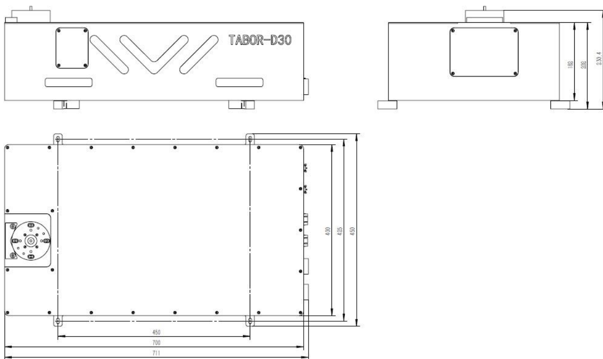
TABOR-D30 激光器尺寸 单位：mm
